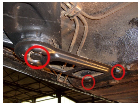
Vordere Achsbefestigung mit Abstützblatt (F). Unter der großen Schraube sitzt ein Gummilager
